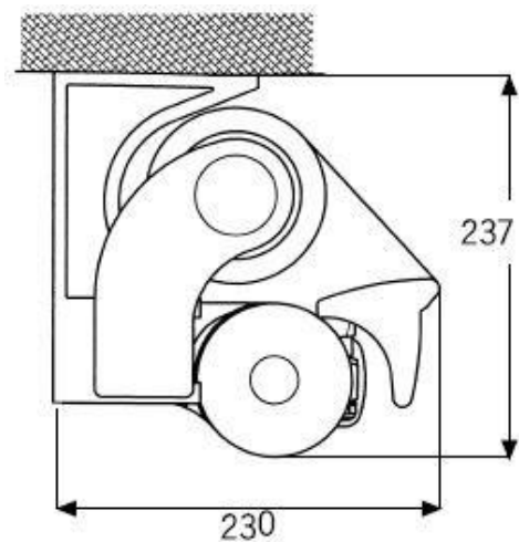
Encombrement plafond
