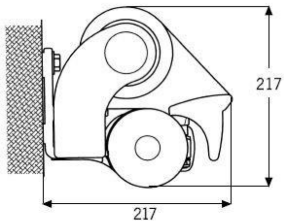
Encombrement face
